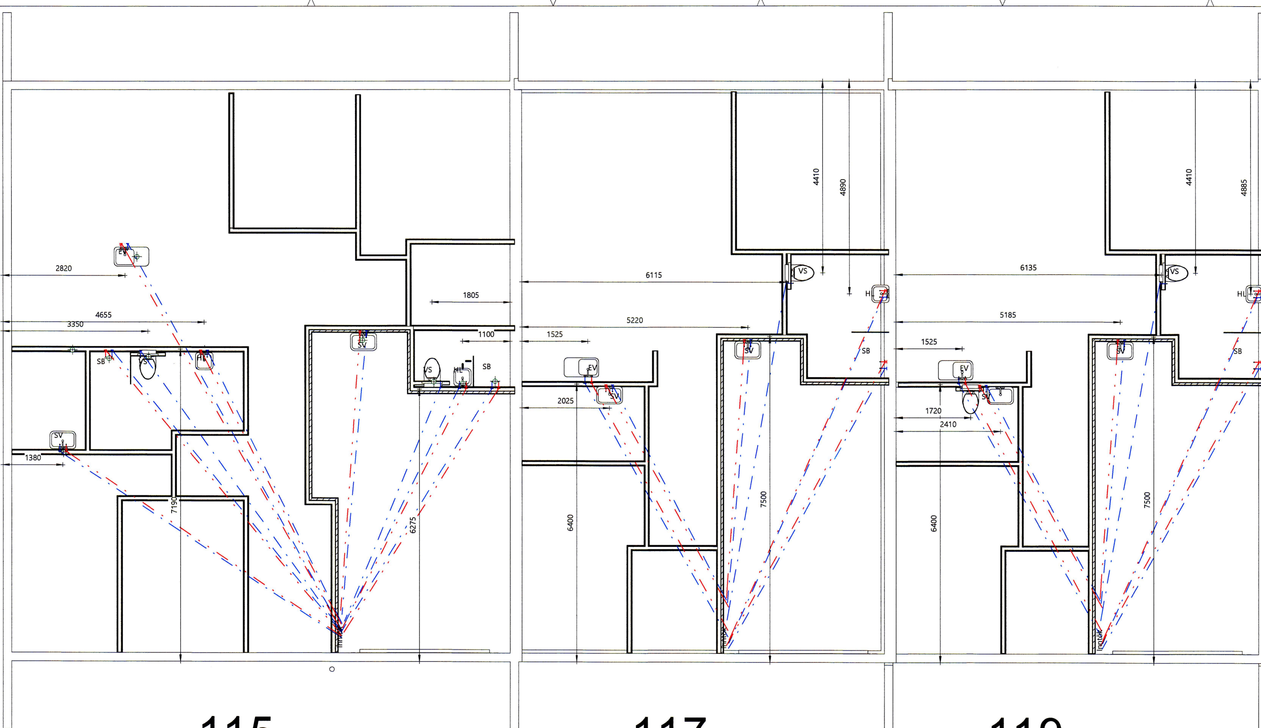
1 Grunnmynd Neysluvatn 115-119 1 : 50
