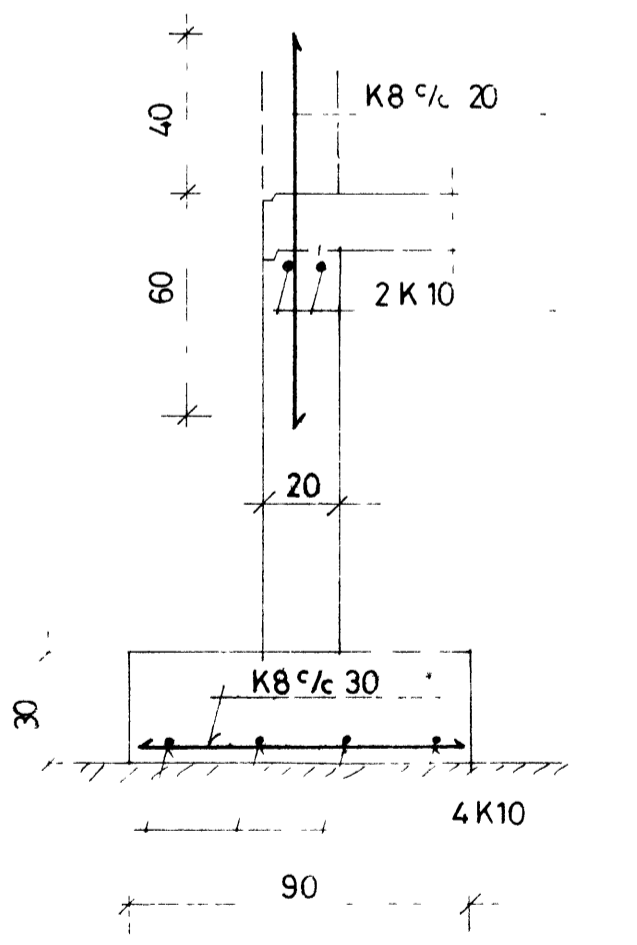
L-L, 1 20
