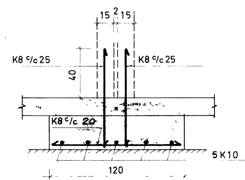
I-I 1 20
