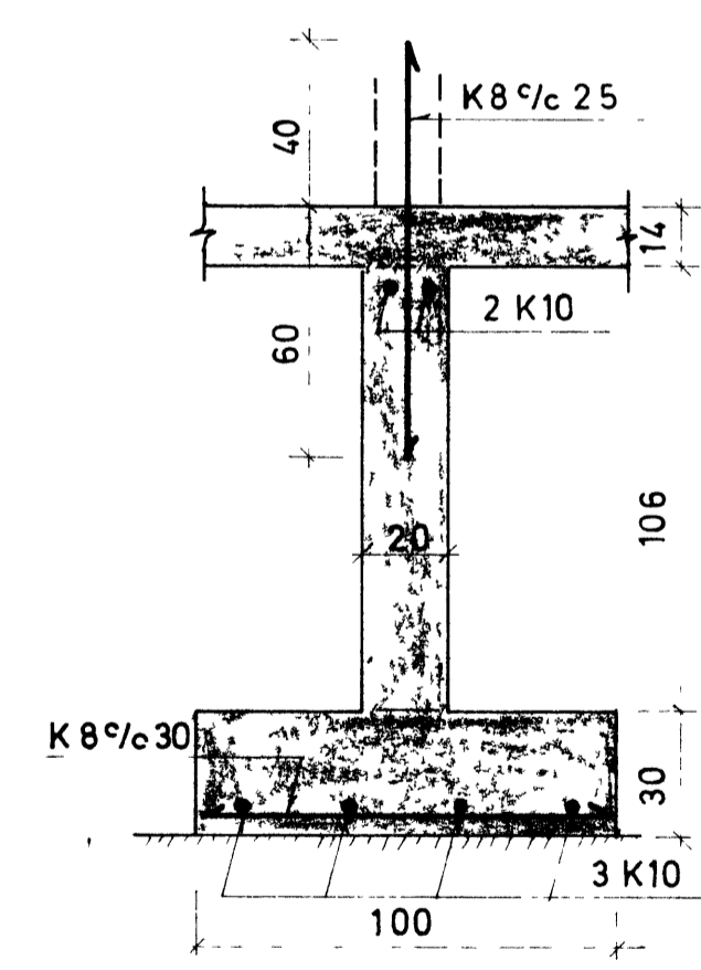
G-G 1 20
