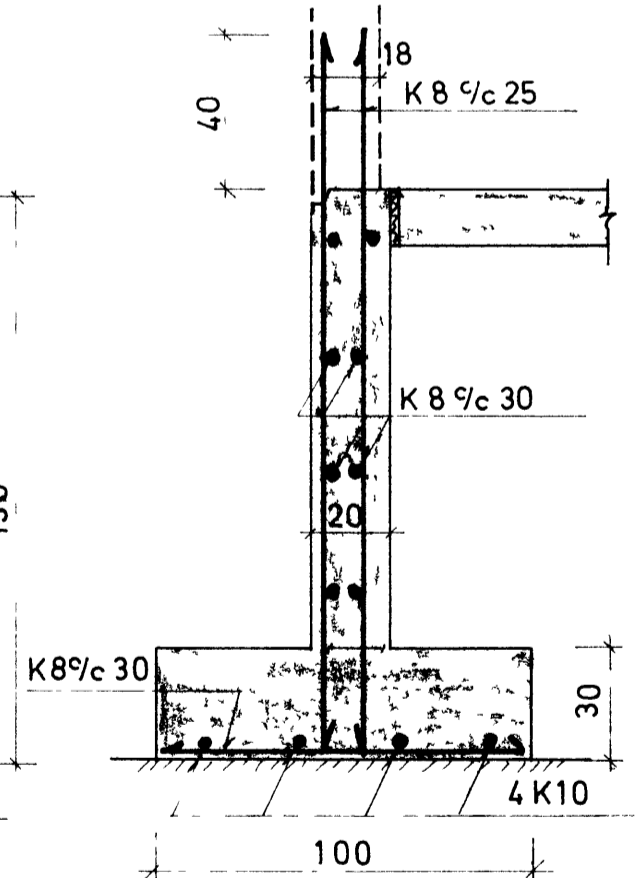
E-E 1 20
