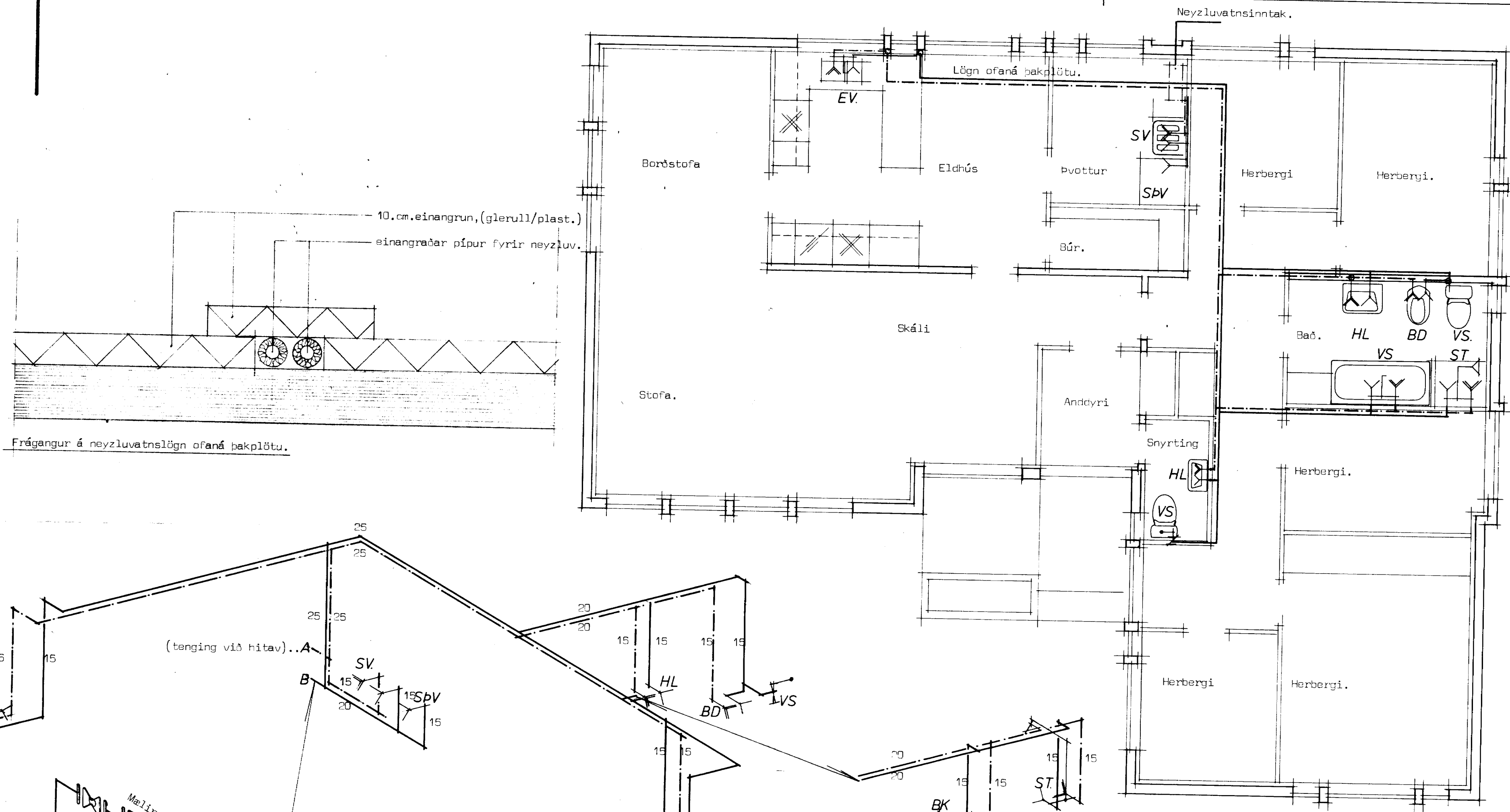
GRUNNMYND m.k.v. 1:50.
