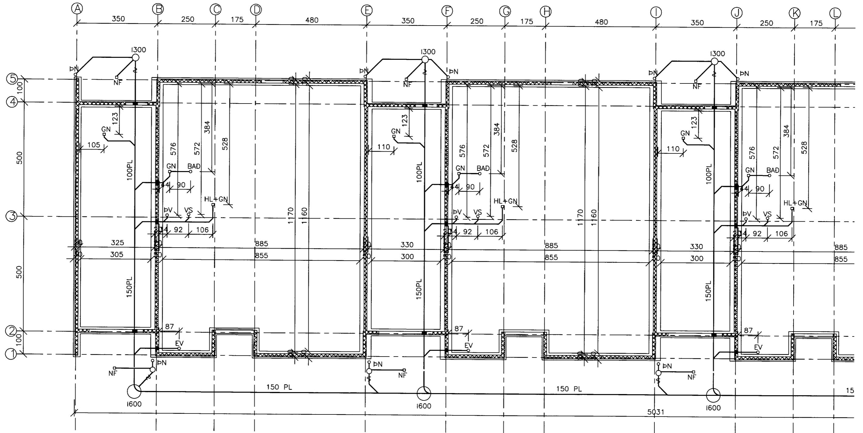
GRUNNMYND M=1:50
