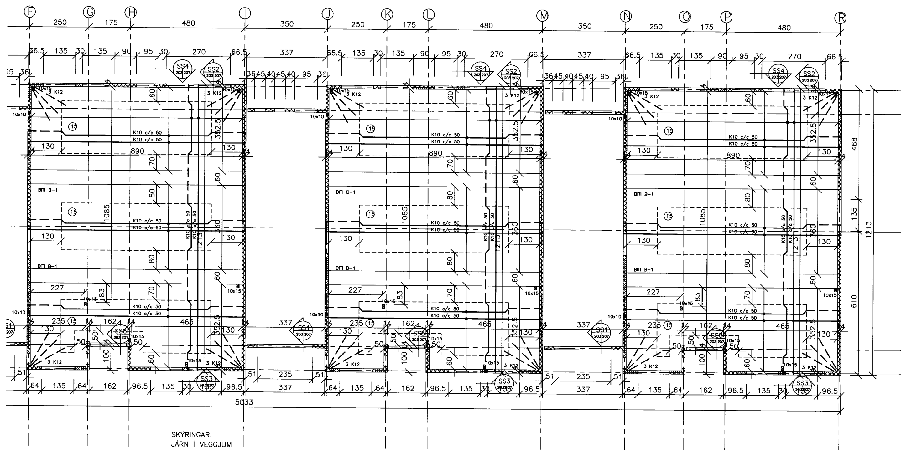
GRUNNMYND M=1:50
