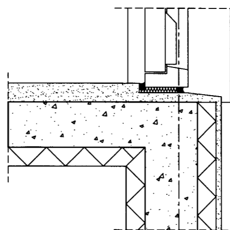
SNID VIÐ ÚTIHURÐ M=1:5
