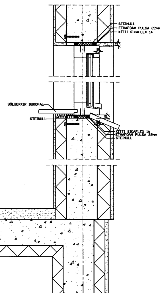
FRÁGANGUR VIÐ GLUGGA M=1:5
