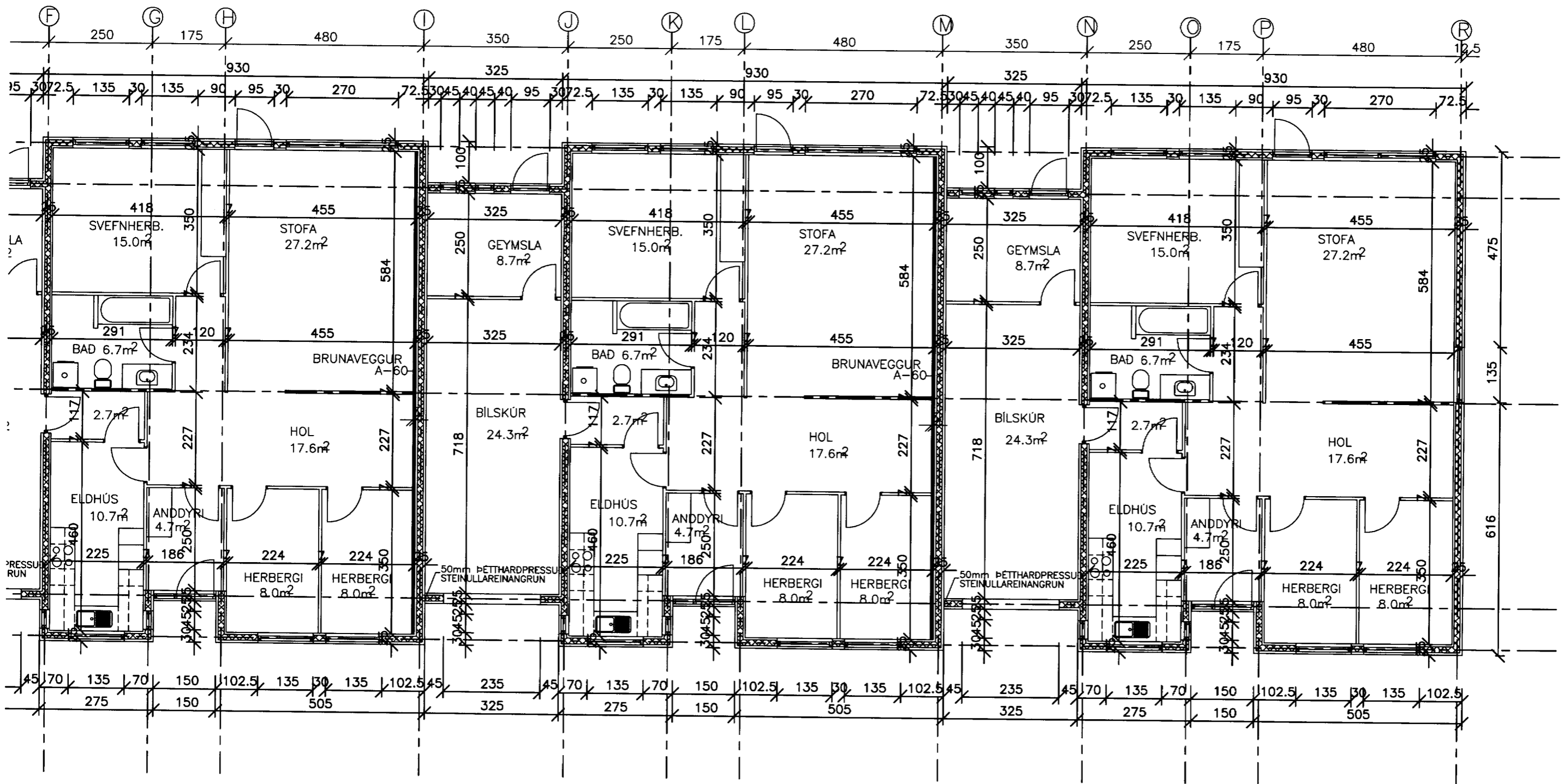
GRUNNMYND M=1:50
