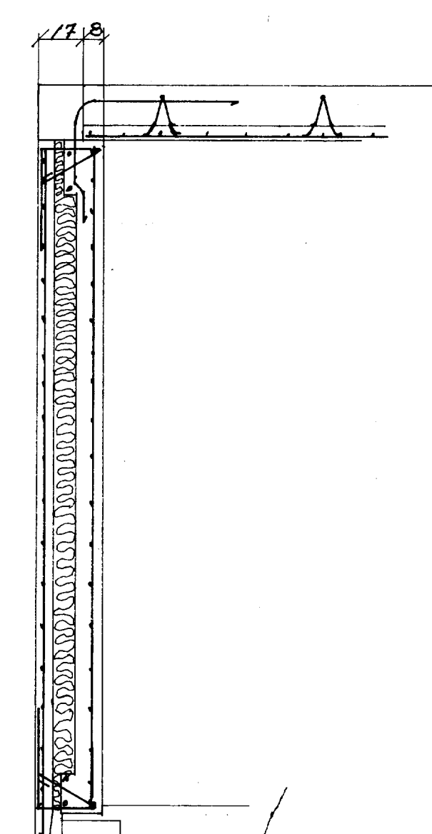
Snid E1: 1:20
