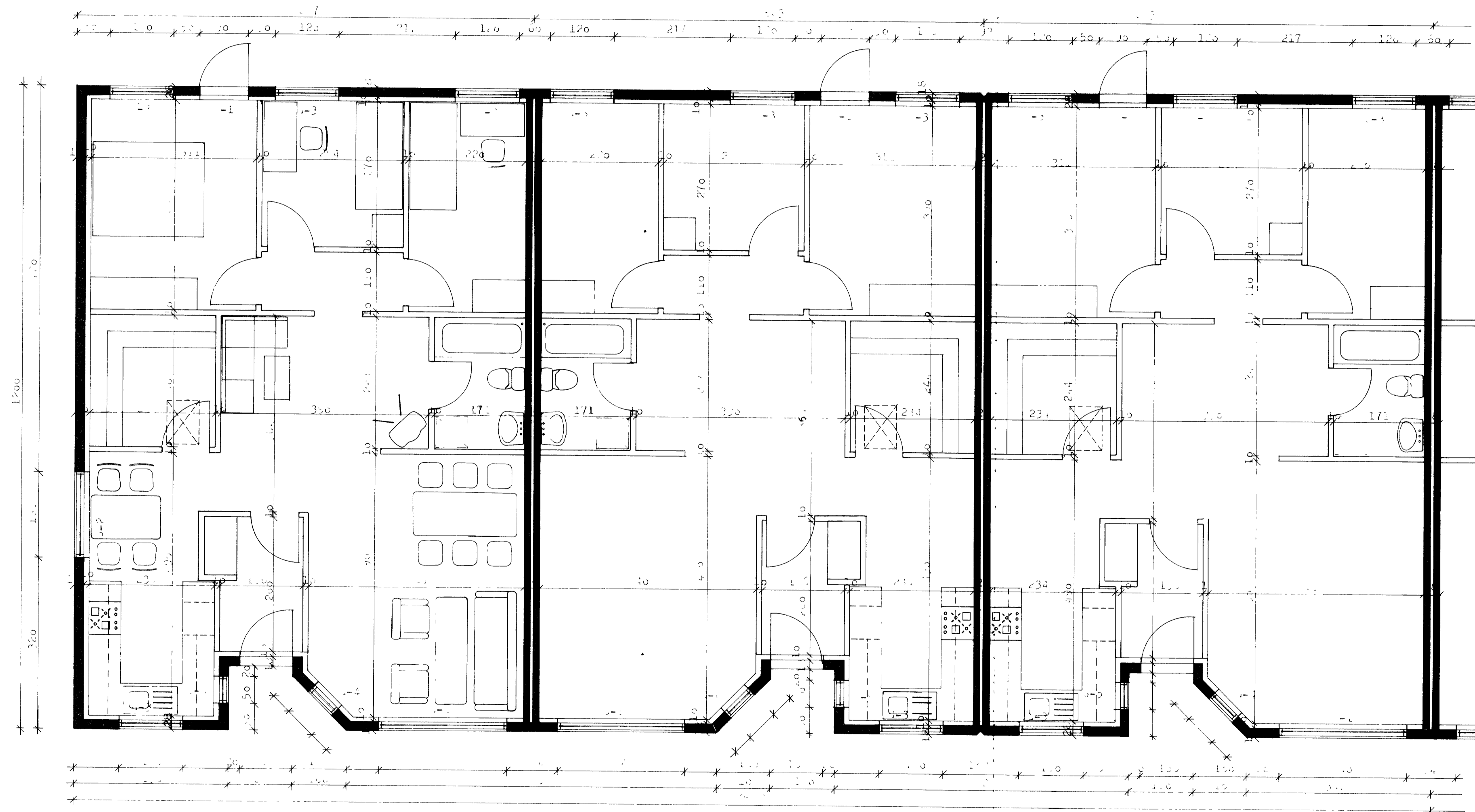
GRUNNMYND Mkv 1:50
