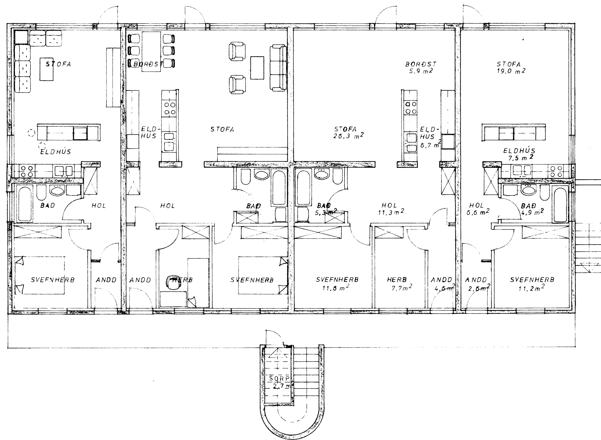
GRUNNMYND 2 HÆÐ 1:100
